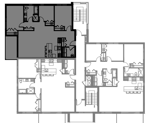
ÉTAGE 1 et 2
