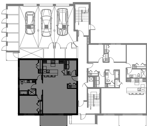
REZ-DE-CHAUSSÉE
